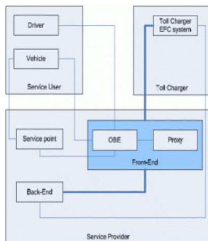
Obrázek 2 – Předpokládaná technic
