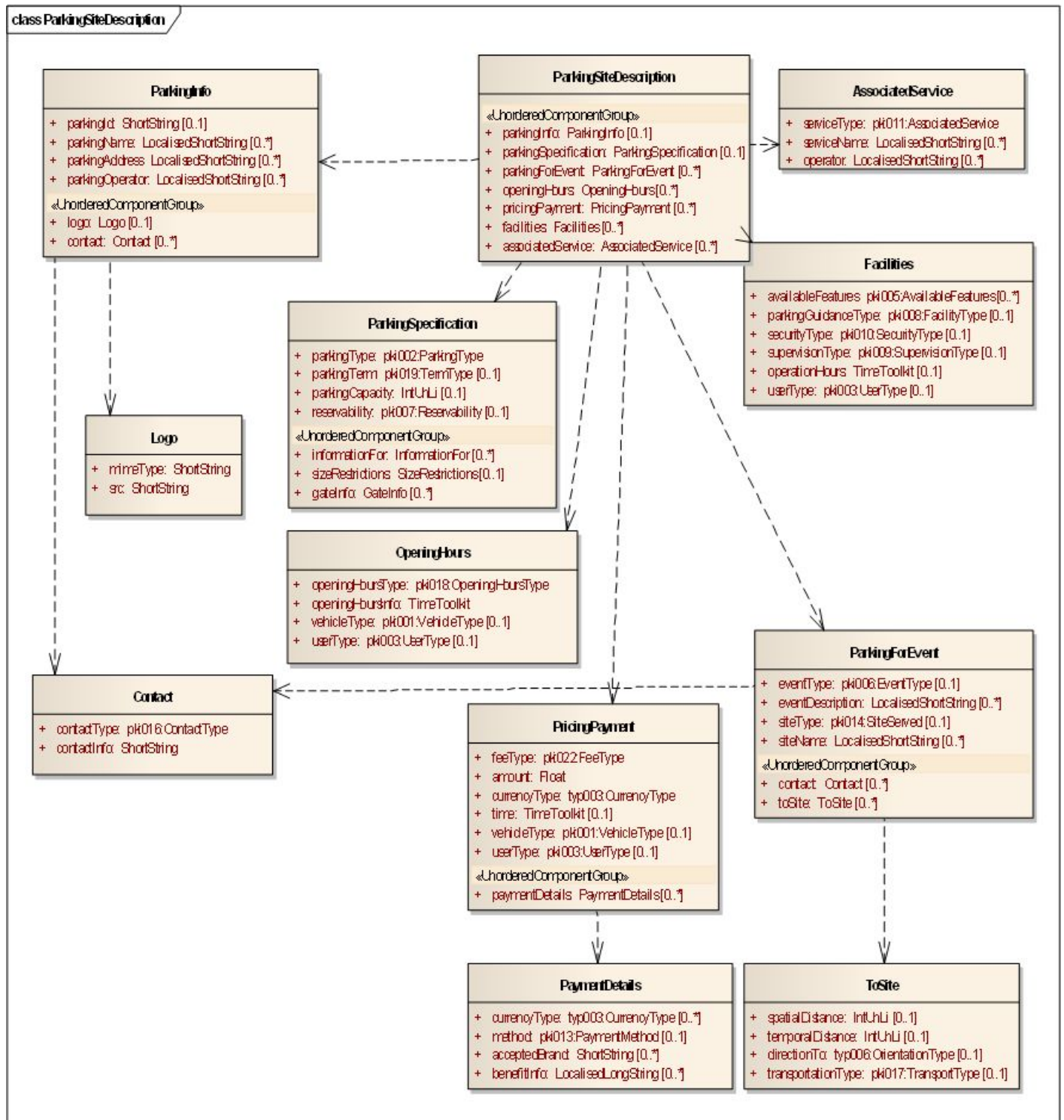
Obrázek 1 - UML model tříd aplikace PKI (obr. 4 normy)
