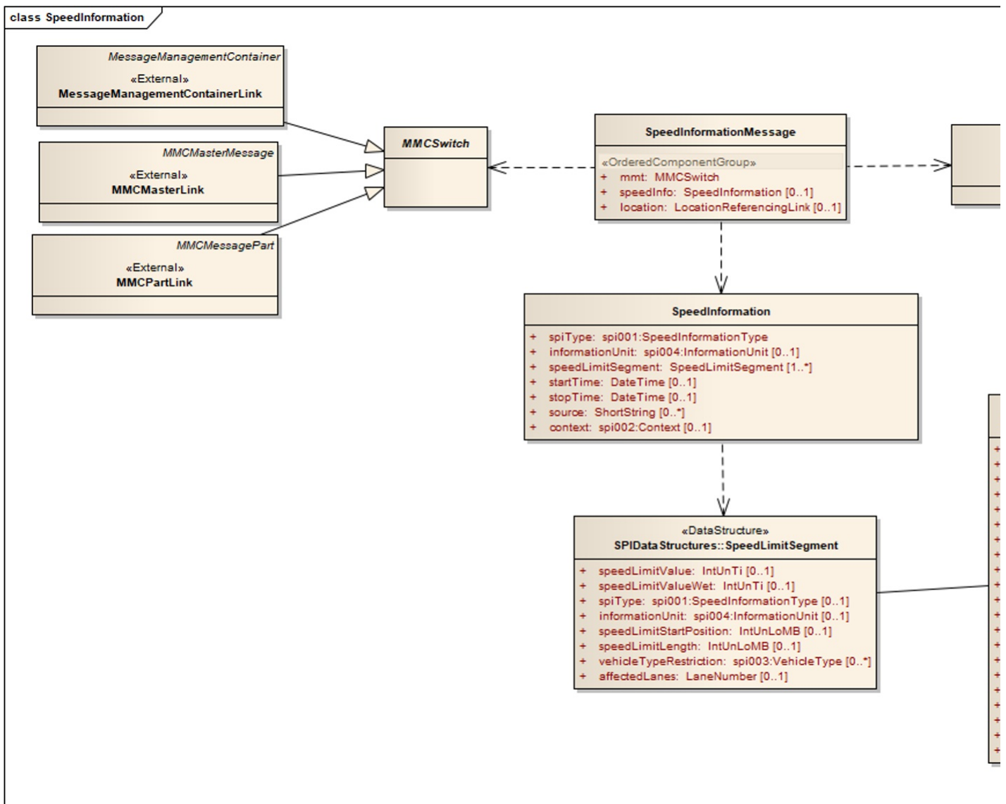
Obrázek 1 - UML model tříd aplikace SPI (obrázek 2 normy)
