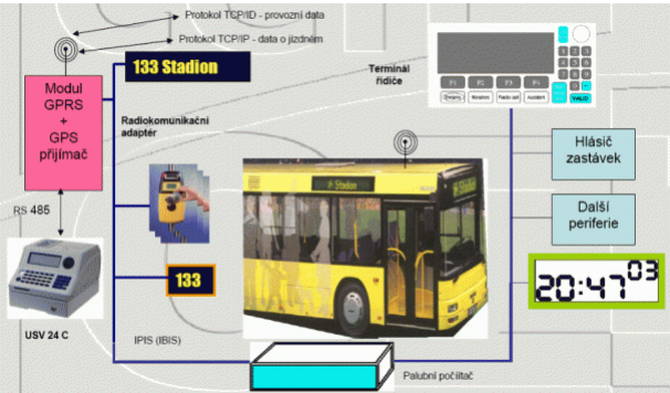
Obrázek 1 – Blokové znázornění informačního a řídicího systému na vozidle veřejné dopravy osob.
