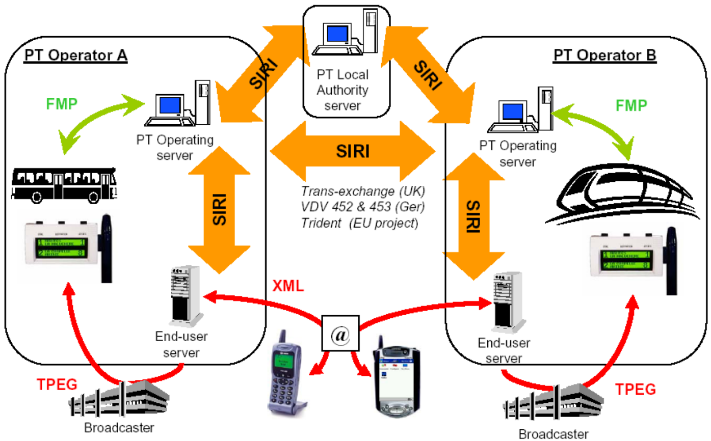
Obrazek 1 – Příklad využití SIRI se znázorněnými komunikačními vazbami v dopravním systému provozovaném dvěma operátory
