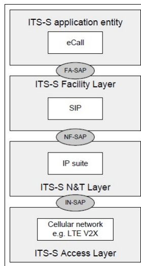
Obrázek 4 - ITS-S protocol stack se SIP (Obrázek 5 normy)
