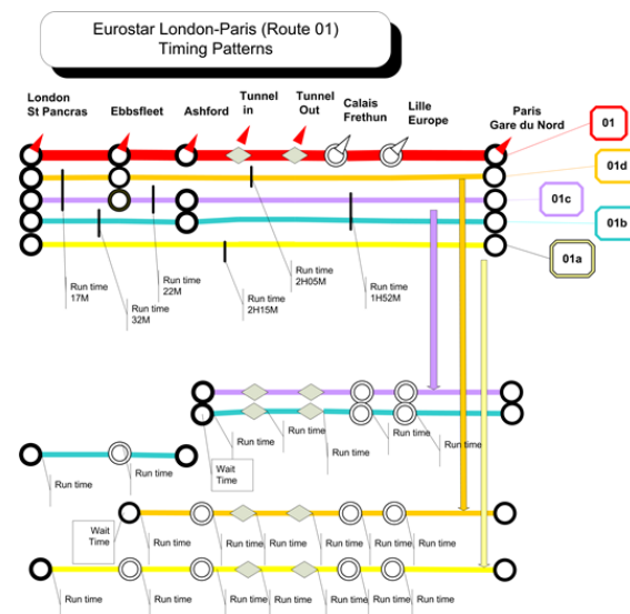
Obrázek 2 – Příklad ukázky časování na železnici, zdroj: NeTEx 1 (obr. 78 normy)
