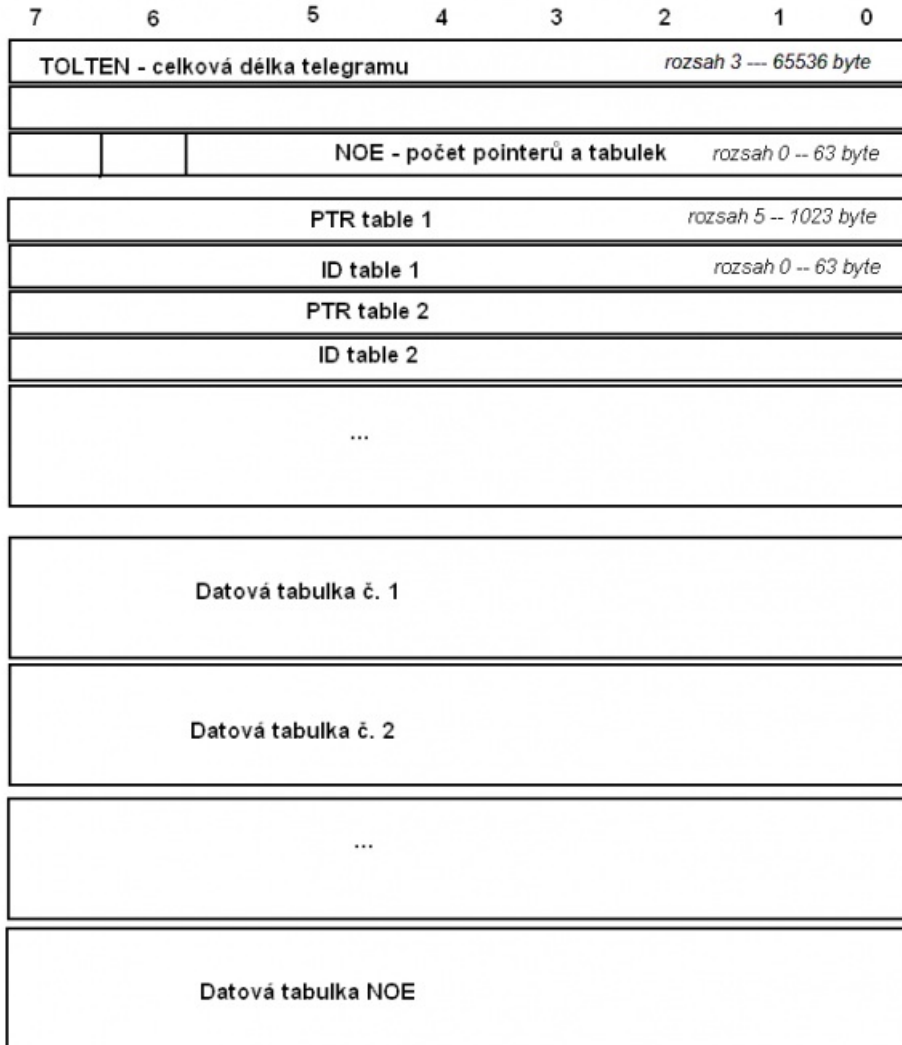
Obrázek 1 - Struktura telegramu
