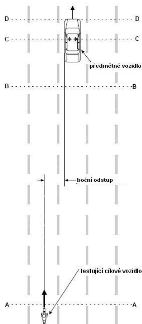
Obrázek 9 – Test – cílové vozidlo předjíždí předmětné vozidlo
