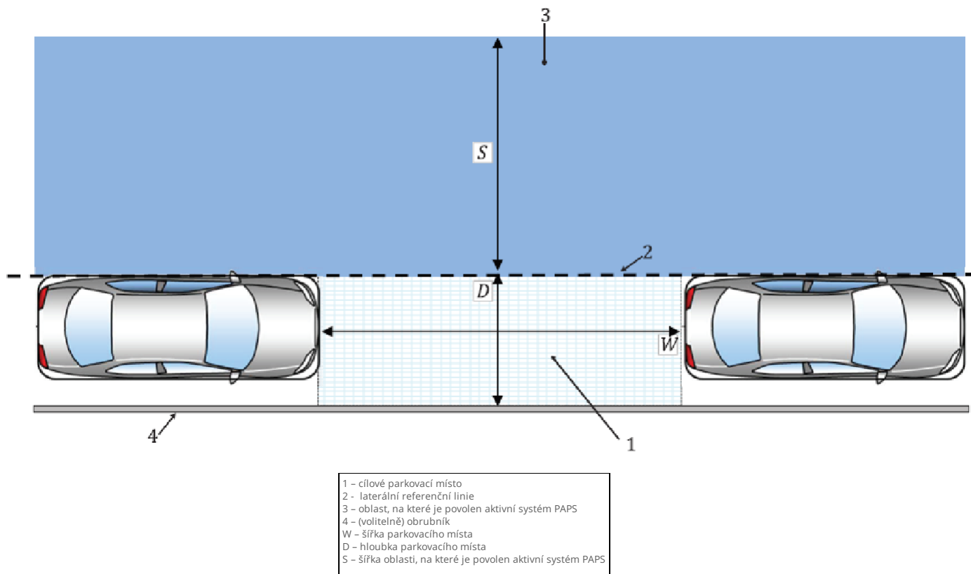
Obrázek 1 - Geometrie podélného parkovacího místa (obr. 1 normy)
