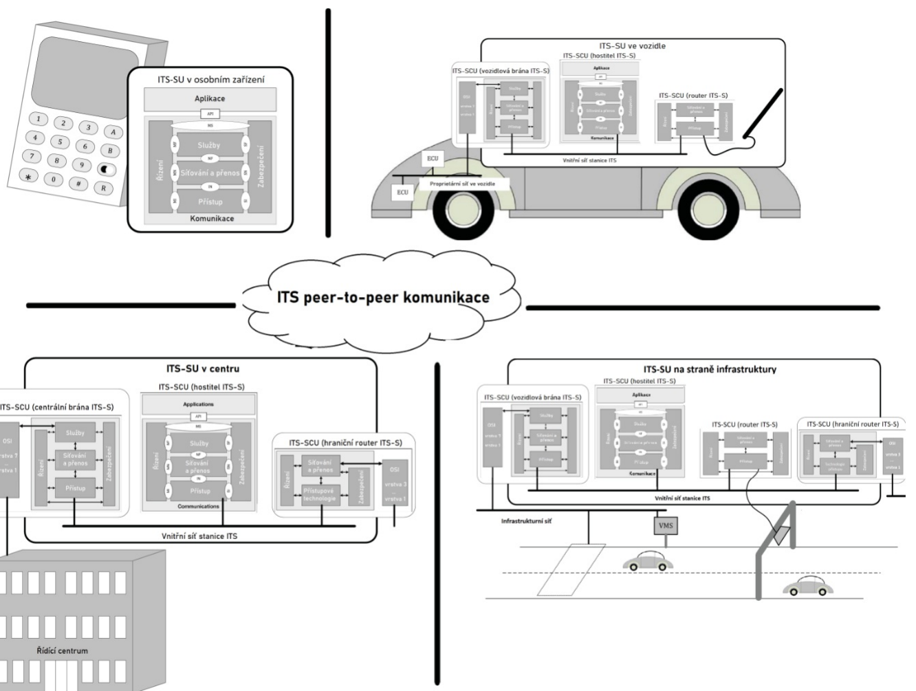
Obrázek 4 - Typická realizace jednotek ITS-SU (obrázek 29 normy)
