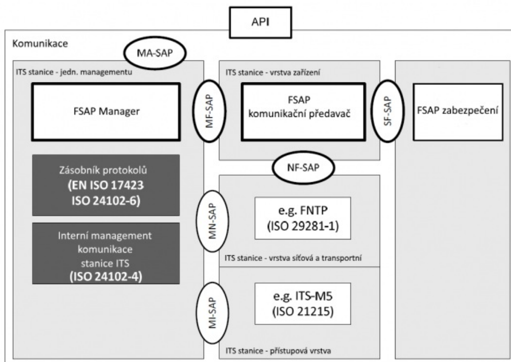
Obrázek 1 – Referenční architektura FSAP (obr. 4 normy)
