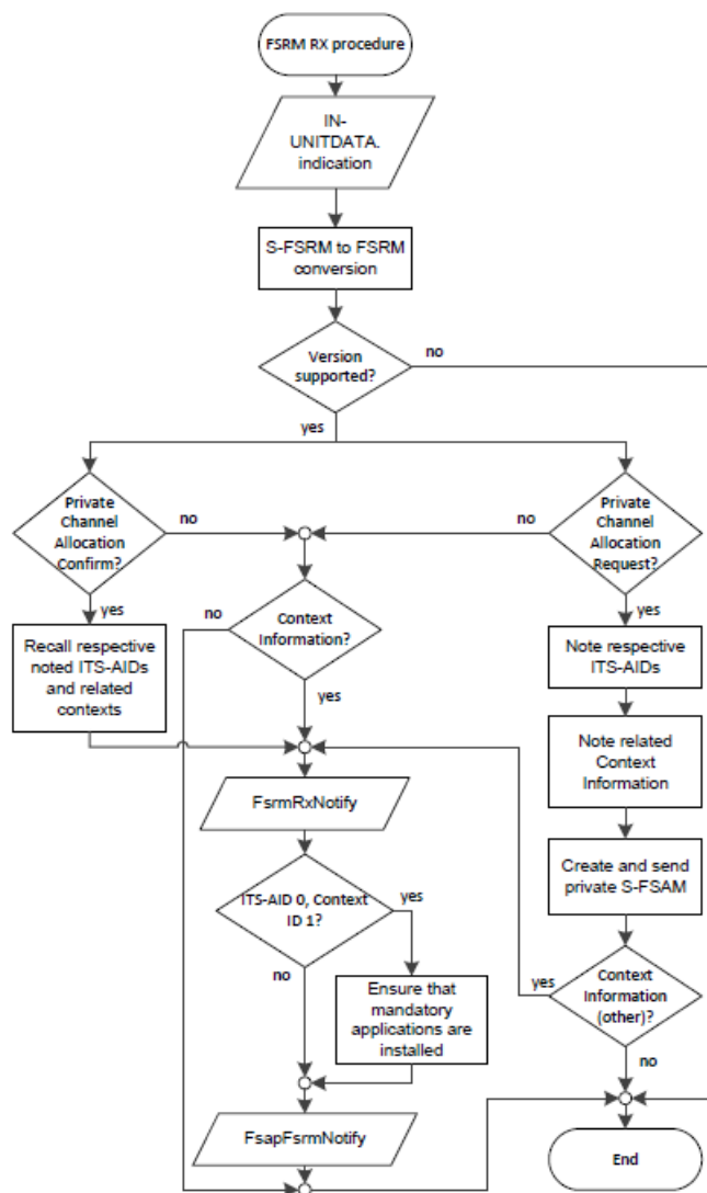
Obrázek 3 – příklad algoritmu zpracování FRSM (obr. 8 normy)
