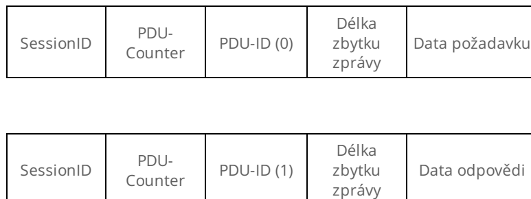
Obrázek 3 – Struktura protokolu RSMP (obr. 7 normy)
