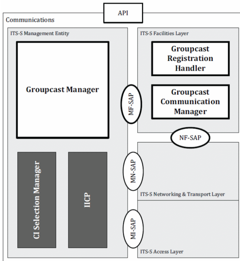
Obrázek 4 - referenční architektura
