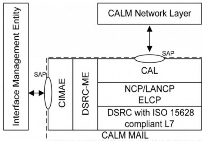
Obrázek 2 – Struktura MAIL
