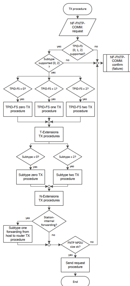
Obrázek 3 - FNTP procedura příjmu dat (obrázek 9 popisované normy)
