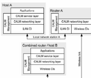
Obrázek 9 – Architektura B (pevná linka host – router, bezdrátové propojení A-B)
