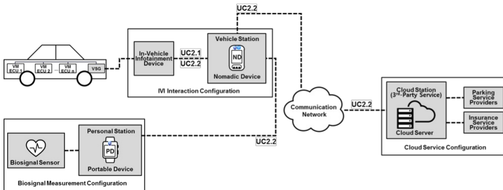
Obrázek 3 — Klaster případů užití 2: Architektura systému (vlevo), demo systém (vpravo), (obrázek č. 4 normy)
