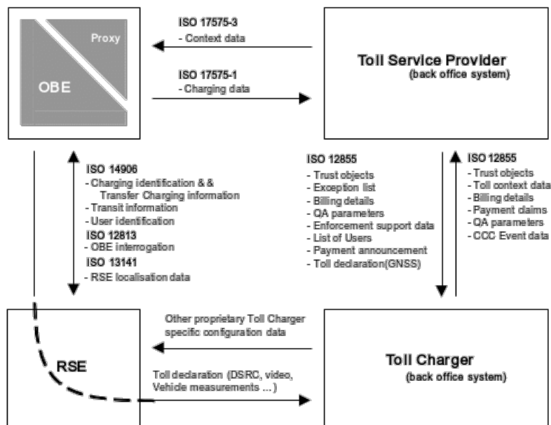
Obrázek 1 – Původní architektura EFC (obr. 3 normy)
