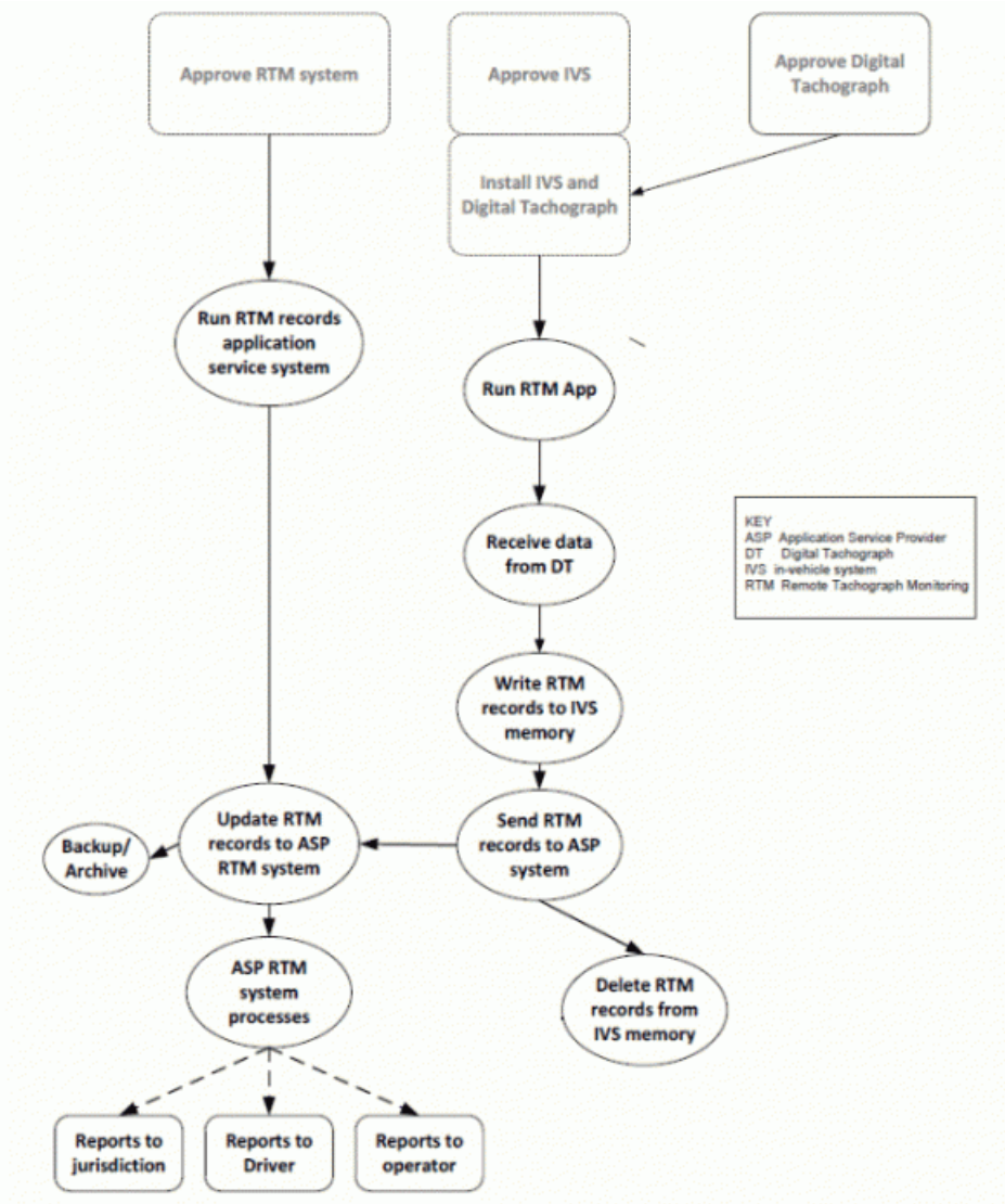
Obrázek 1 – Procesní diagram TARV RTM (Obrázek 9 normy)
