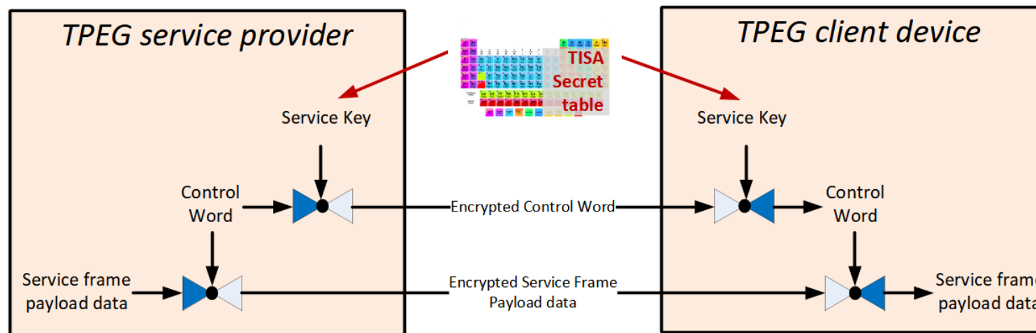
Obrázek 1 - princip šifrování v režimu 1 (obrázek 1 normy)
