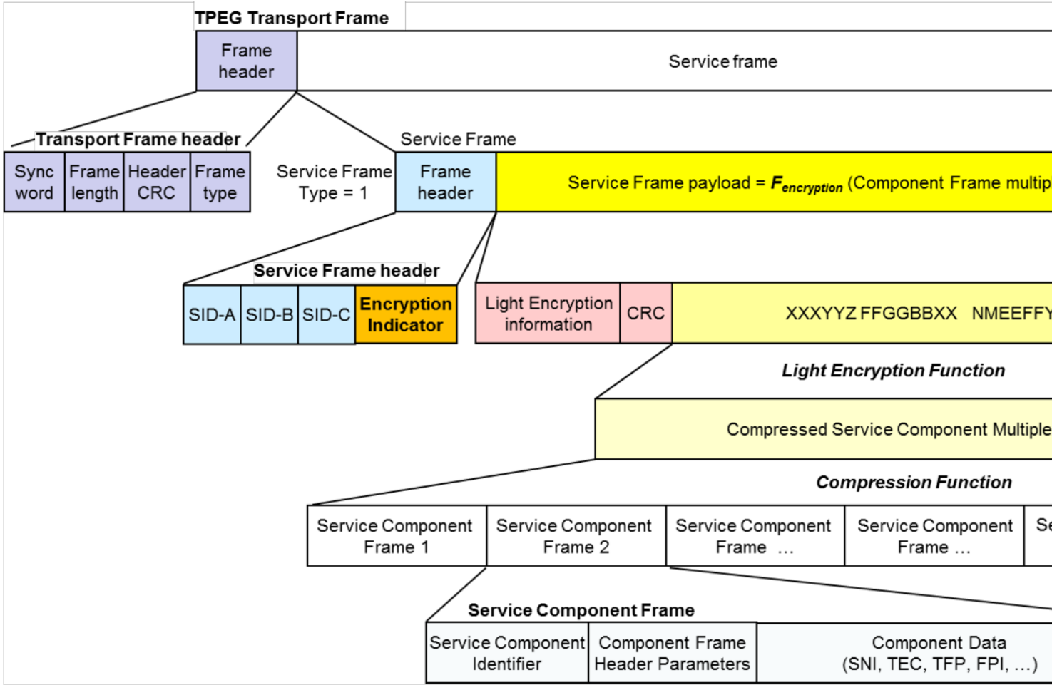
Obrázek 2 - Složení, komprese, šifrování a rámec pro TPEG LTE (obrázek 7 normy)
